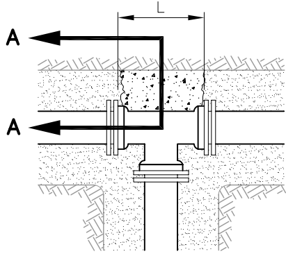
TEE
